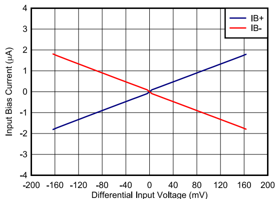
図 6-14. 入力バイアス電流と差動入力電圧の関係
