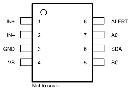
図 5-2. DDF パッケージ 8 ピン SOT-23 (上面図)
