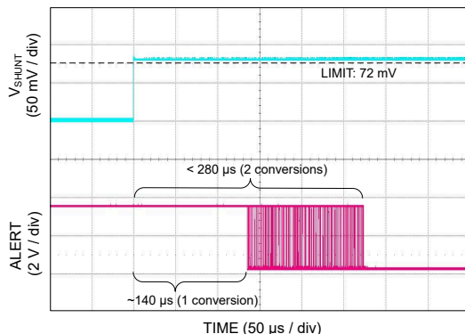
図 8-3. アラート応答 ( t_{CT} = 140\mu s )
