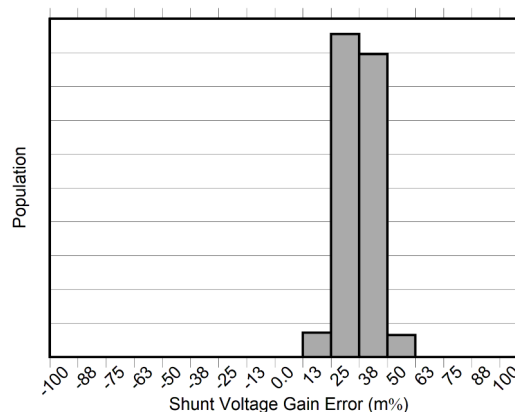
図 6-7. シャント電圧のゲイン誤差の製造分布
