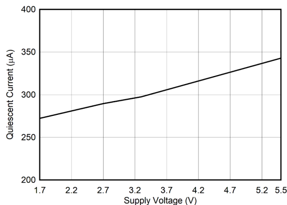
図 6-19. 静止電流と電源電圧との関係
