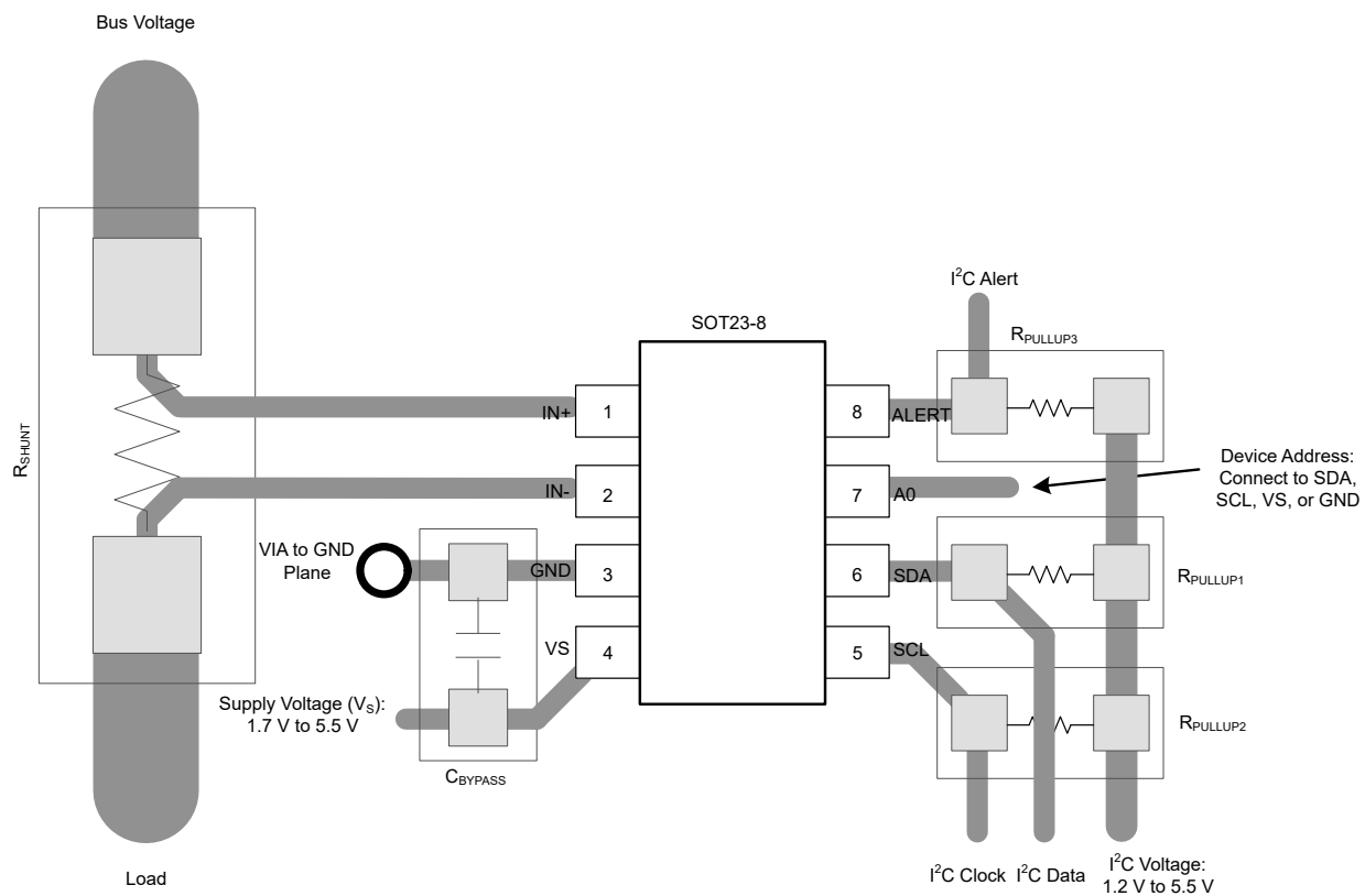
図 8-6. INA236 DDF のレイアウト例 (ハイサイド)
