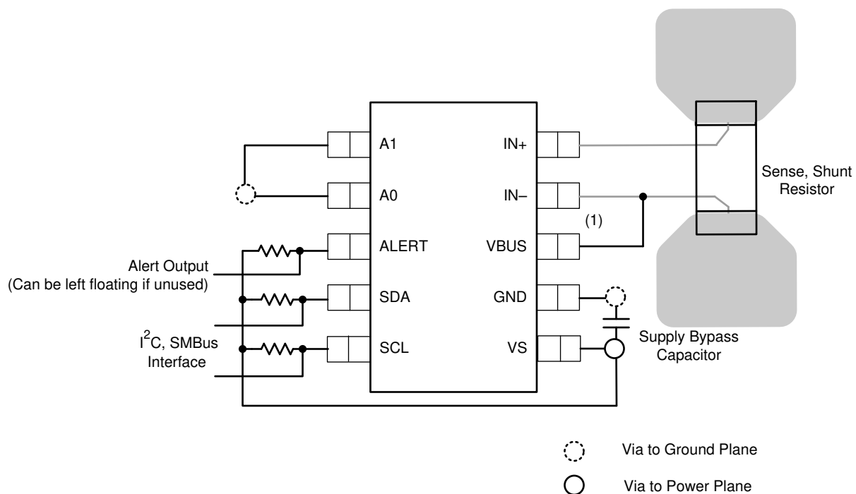
図 7-4. INA233 Layout Example
