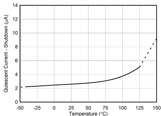
図 6-16. シャットダウン時の静止電流と温度との関係
