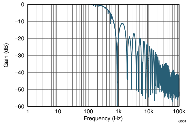
図 6-2. 周波数応答
