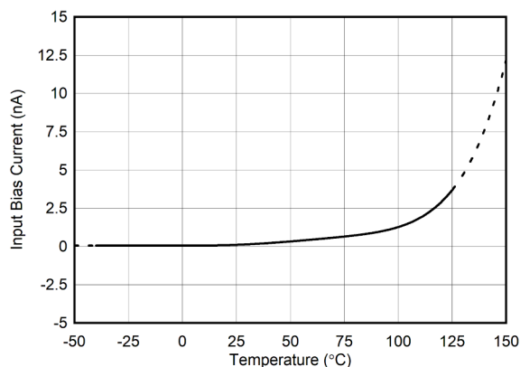
図 6-11. 入力バイアス電流と温度との関係
