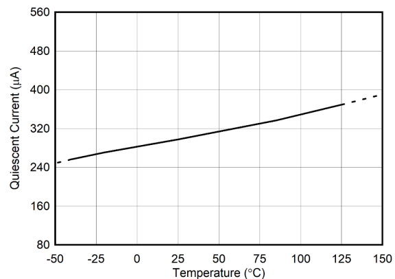
図 6-13. 静止電流と温度との関係
