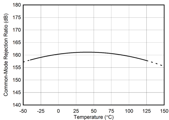
図 6-4. シャント入力 CMRR と温度との関係
