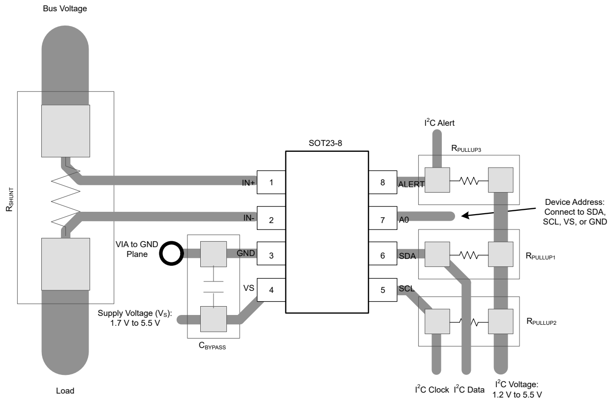
図 8-5. INA232 DDF のレイアウト例 (ハイサイド)
