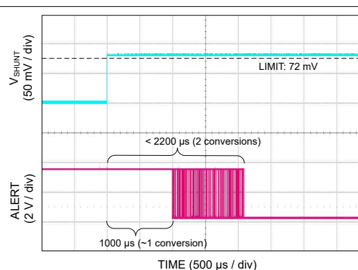
図 8-4. アラート応答 ( t_{CT} = 1.1\text{ms} )
