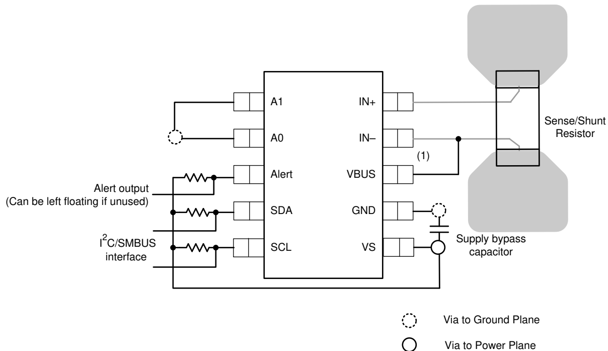
8-4. INA226-Q1 Layout Example
