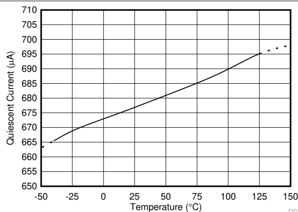
図 6-25. 静止電流と温度との関係 (INA181-Q1)
