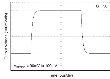
图 15. Step Response
