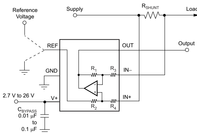
概略回路図
