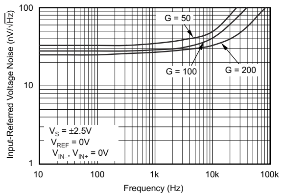
図 6-12. 入力換算電圧ノイズと周波数との関係
