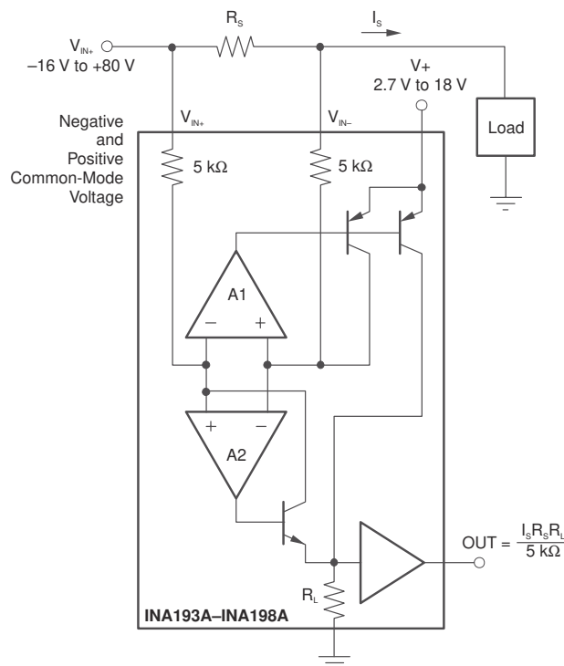
簡略回路図
