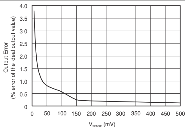
FIG 6-5. Output Error vs Vsense
