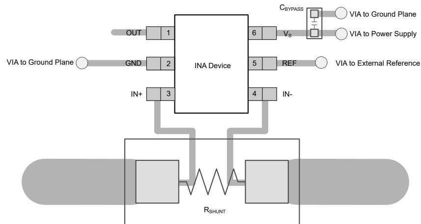
図 7-3. INA187-Q1 SOT-23 6 ピン (DBV) パッケージの推奨レイアウト
