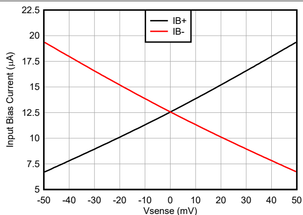
図 5-14. INA187-Q1 ゲイン = 50V/V、入力バイアス電流と V_{\text{SENSE}} との関係
