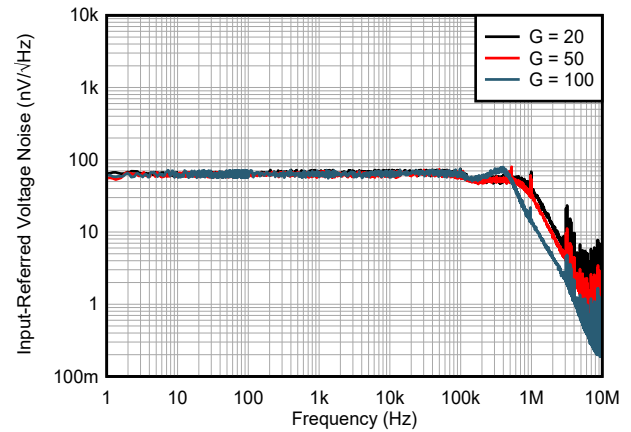
図 5-22. 入力換算ノイズと周波数との関係
