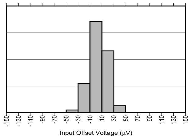
図 5-1. INA187-Q1 入力オフセット電圧の製品分布
