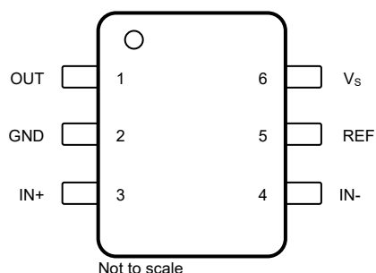
図 4-1. INA187-Q1 : DBV パッケージ 6 ピン SOT-23 上面図
