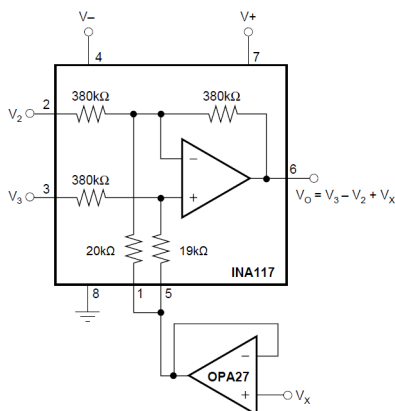
図 7-10. Summing V X in Output
