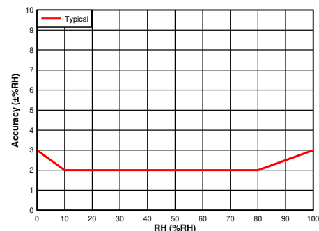
RH 精度 (T A = 30°C)
