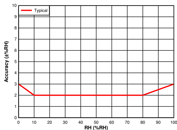
RH (相対湿度) の精度 (T A = 30°C)
