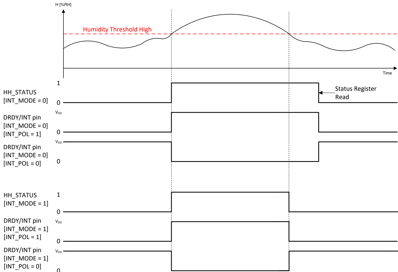
図 7-5. スレッシュールド上の割り込み - 湿度 HIGH
