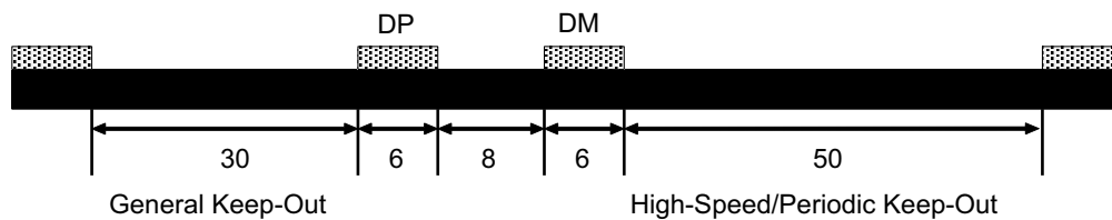
図 9-3. USB2 差動信号の間隔 (mil)
