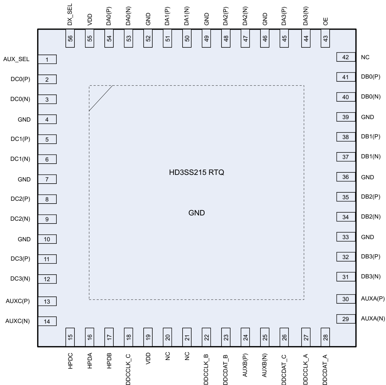
図 6-2. 56-Pin QFN RTQ Package (Top View)
