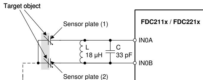
図 8-2. 差動センサ構成
