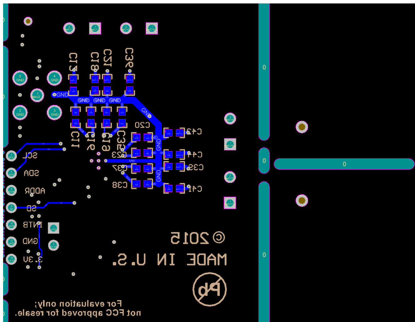
図 7-12. Example PCB Layout: Bottom Layer (Signal)
