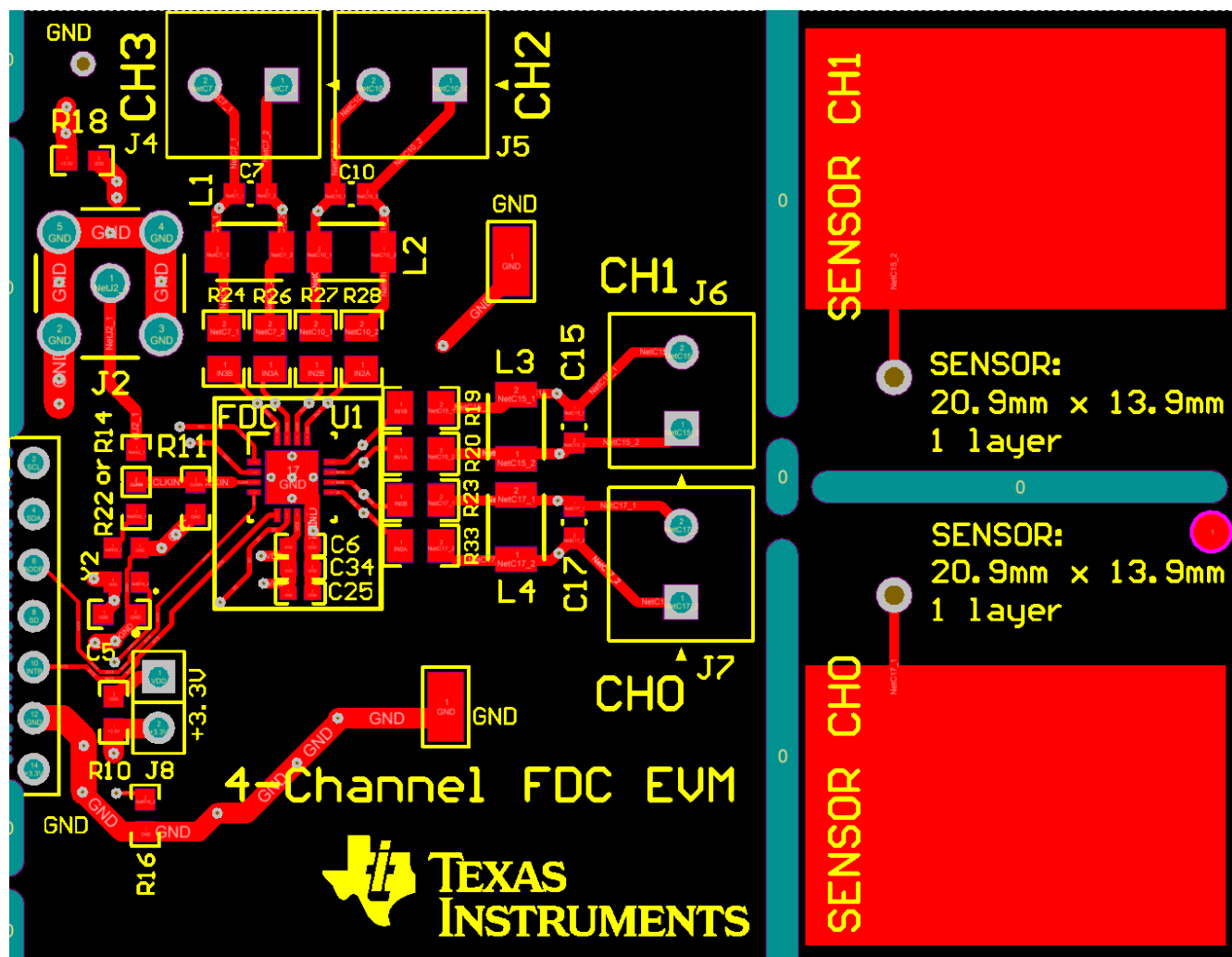
図 7-9. Example PCB Layout: Top Layer (Signal)
