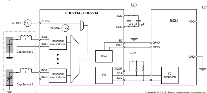
概略回路図
