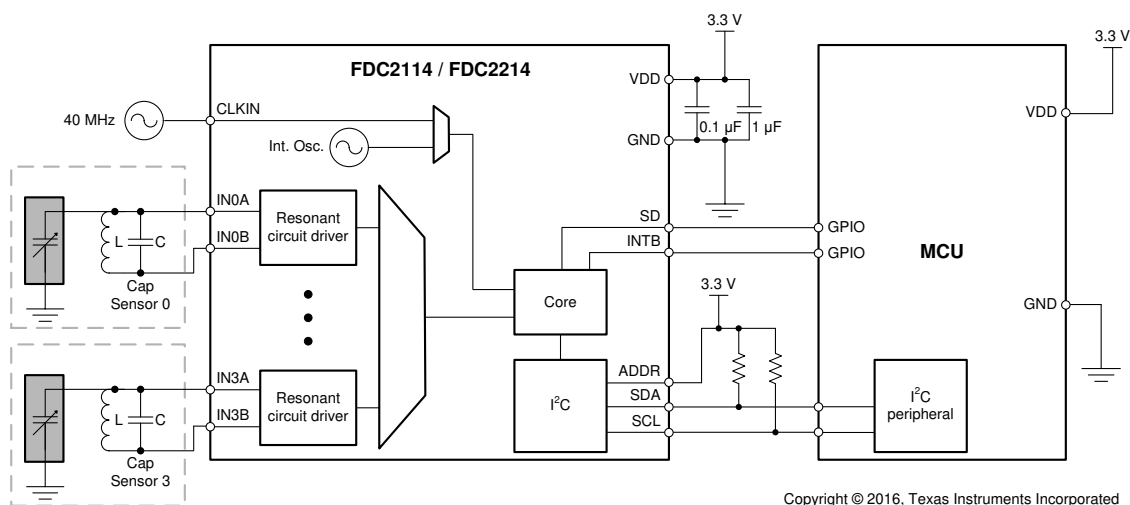
概略回路図
