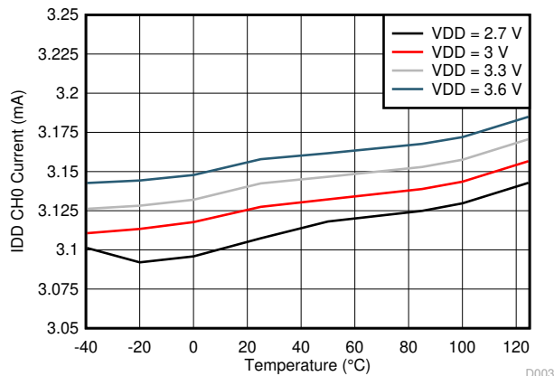
図 6-2. アクティブ モードの IDD と温度との関係
