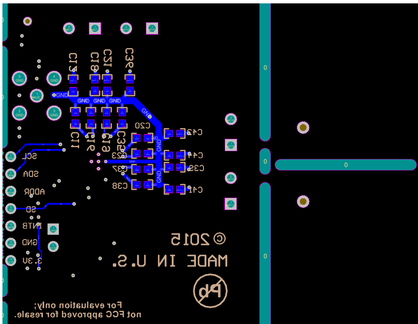
図 8-13. PCB レイアウトの例：最下層 (信号)
