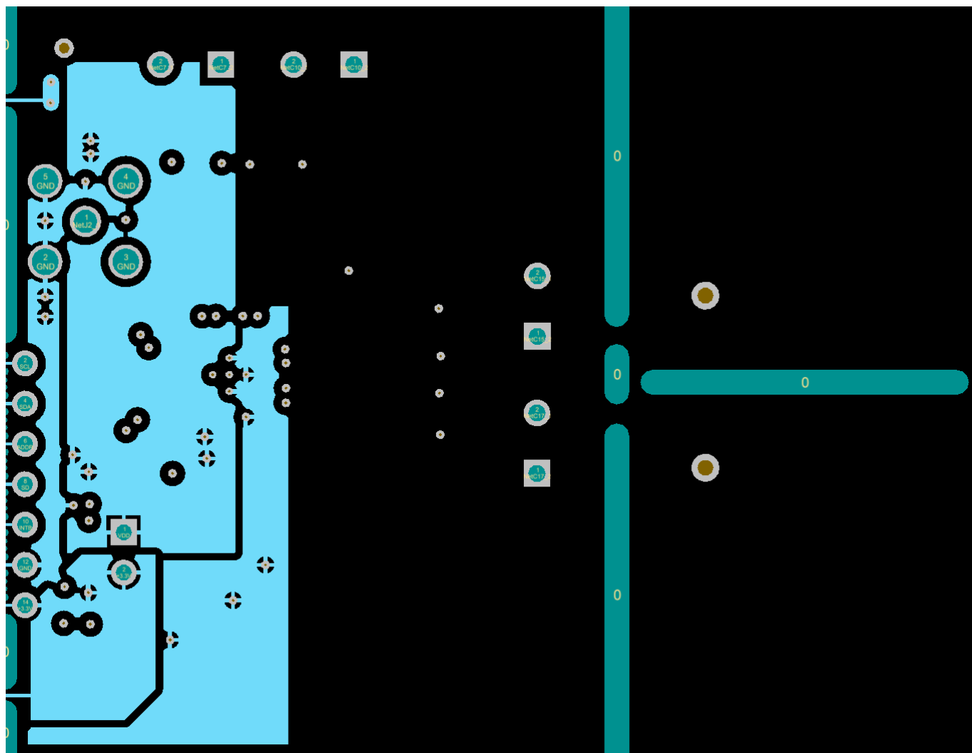
図 8-12. PCB レイアウトの例 : 中間層 2 (電源)
