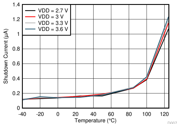
図 6-6. シャットダウン モードの IDD と温度との関係
