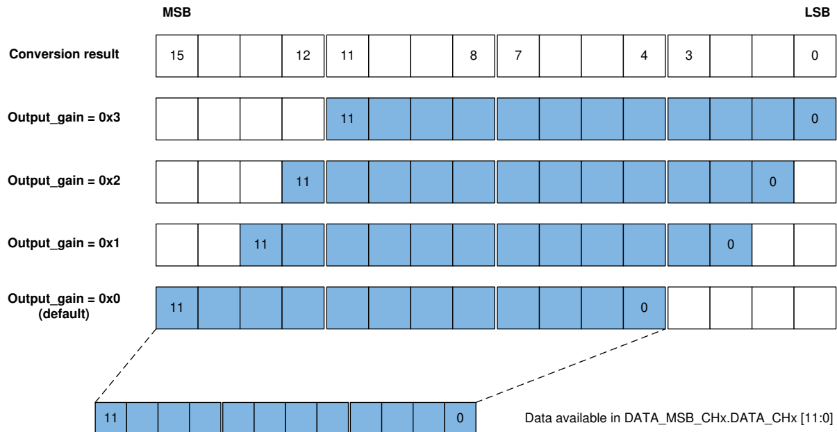
図 7-6. 変換データ出力のゲイン
