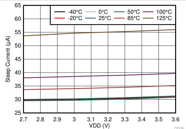
図 6-5. スリープ モードの IDD と VDD との比較
