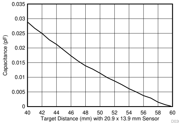
図 8-6. FDC2212/FDC2214 : 容量とターゲット距離の関係 (40~60mm)
