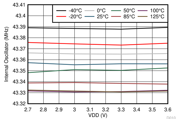
図 6-9. 内部発振器周波数と VDD との関係
