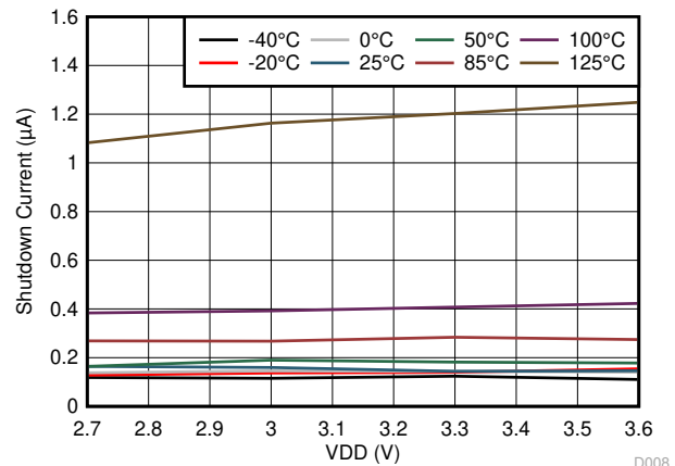
図 6-7. シャットダウン モードの IDD と VDD との関係
