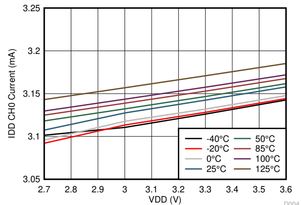
図 6-3. アクティブ モードの IDD と VDD との関係
