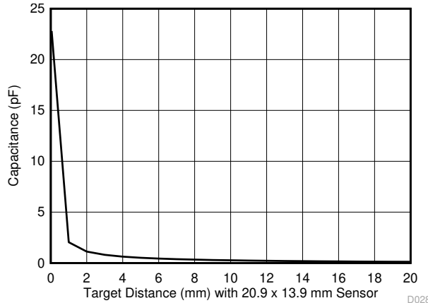
図 8-4. FDC2212/FDC2214 : 容量とターゲット距離の関係 (0~20mm)
