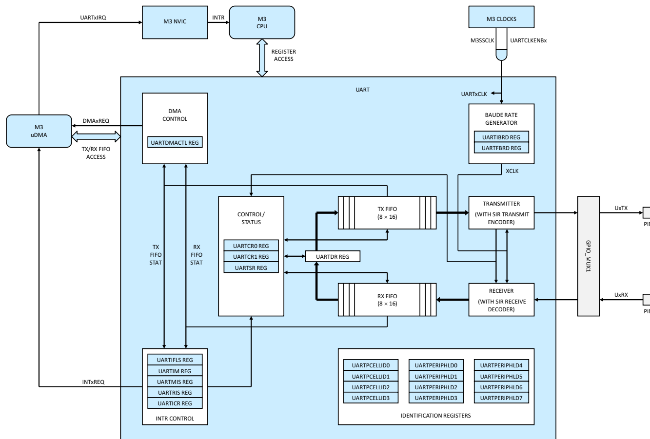
图 7-31. UART
