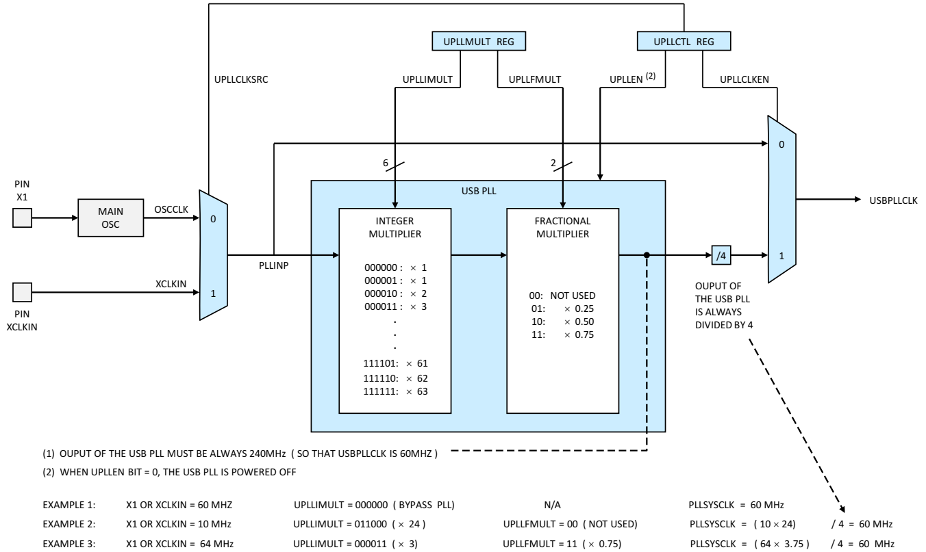
图 8-9. USB PLL
