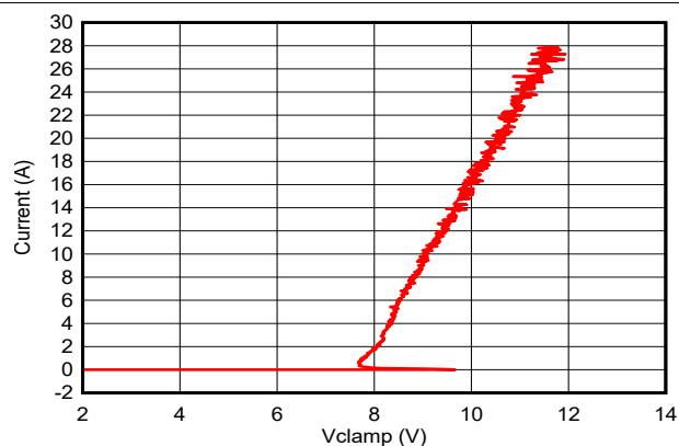
図 5-6. Positive TLP Curve
