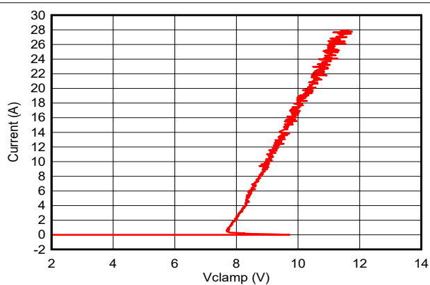
图 5-7. Negative TLP Curve
