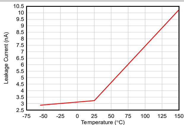
図 5-3. リーク電流と温度との関係
