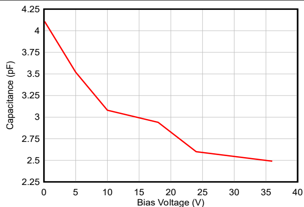
図 5-2. 静電容量とバイアス電圧との関係
