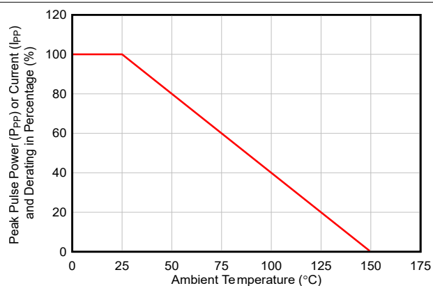
図 5-4. ピーク パルス電力のディレーティング曲線
