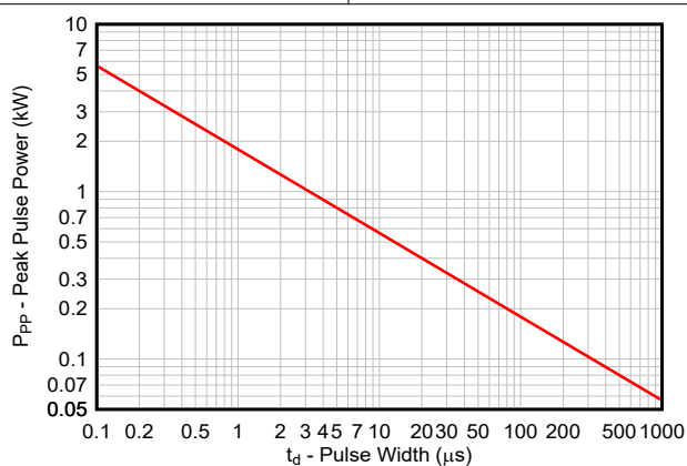
図 5-5. パルス電力の定格曲線
