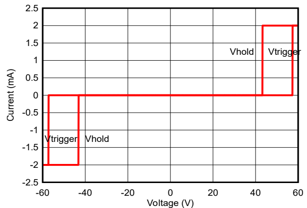
図 5-2. DC I-V Curve
