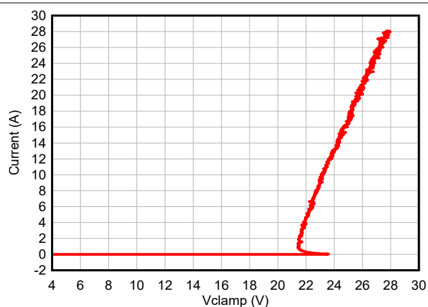
図 5-6. Positive TLP Curve
