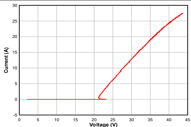
図 5-4. Negative TLP Curve
