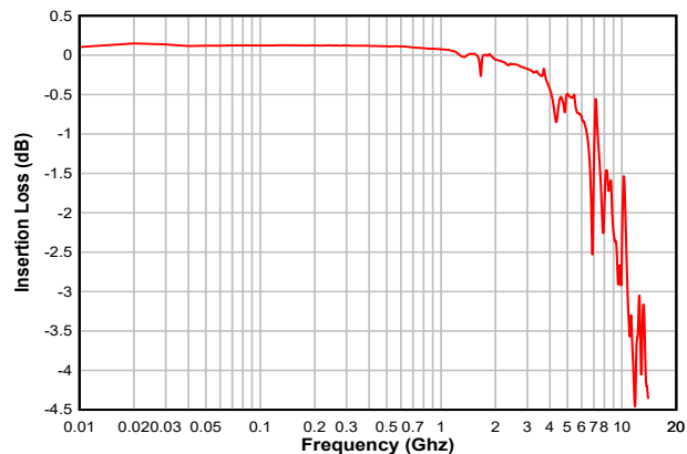
図 5-8. Insertion Loss
