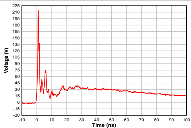
図 5-6. +8kV Clamped IEC Waveform
