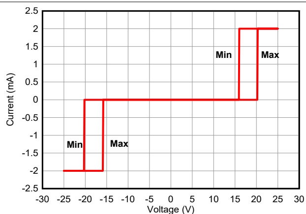
図 5-7. DC Voltage Sweep I-V Curve
