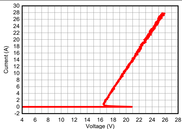
図 5-6. Negative TLP Curve
