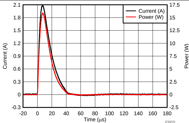
图 5. IEC 61000-4-5 Surge Waveform ( t_p=8/20\text{ }\mu\text{s} )
