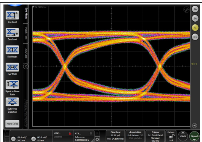
图 14. HDMI 2.0 6 Gbps Eye Diagram with ESD224
