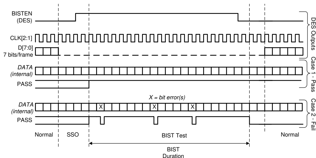
图 7-14. BIST Waveforms
