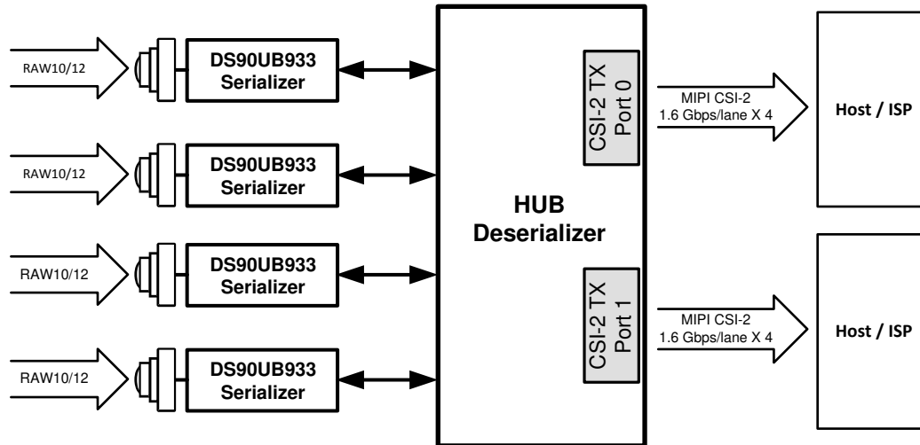
図 6-10. Four DS90UB933-Q1 Sensor Data Onto CSI-2 Over 2 Ports
