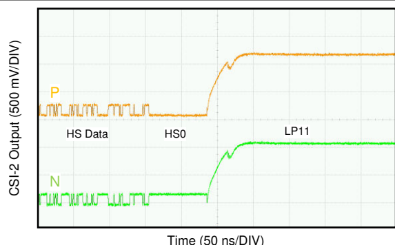
図 8-11. CSI-2 End of Transmission (EoT)
