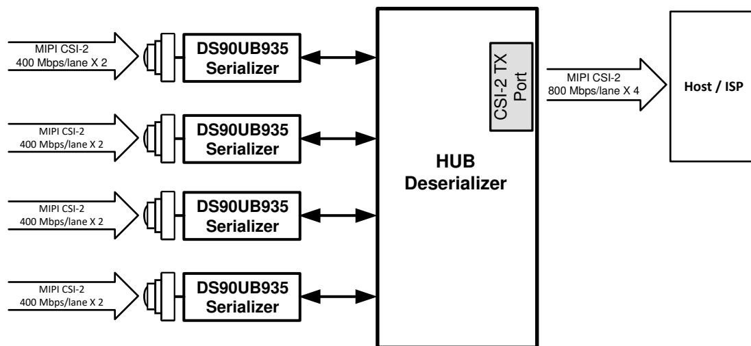
図 8-12. Four DS90UB935-Q1 Sensor Data Onto CSI-2
