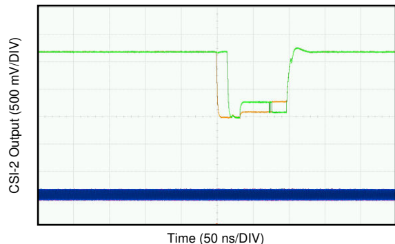
図 8-9. CSI-2 DATA and Continuous CLK Output
