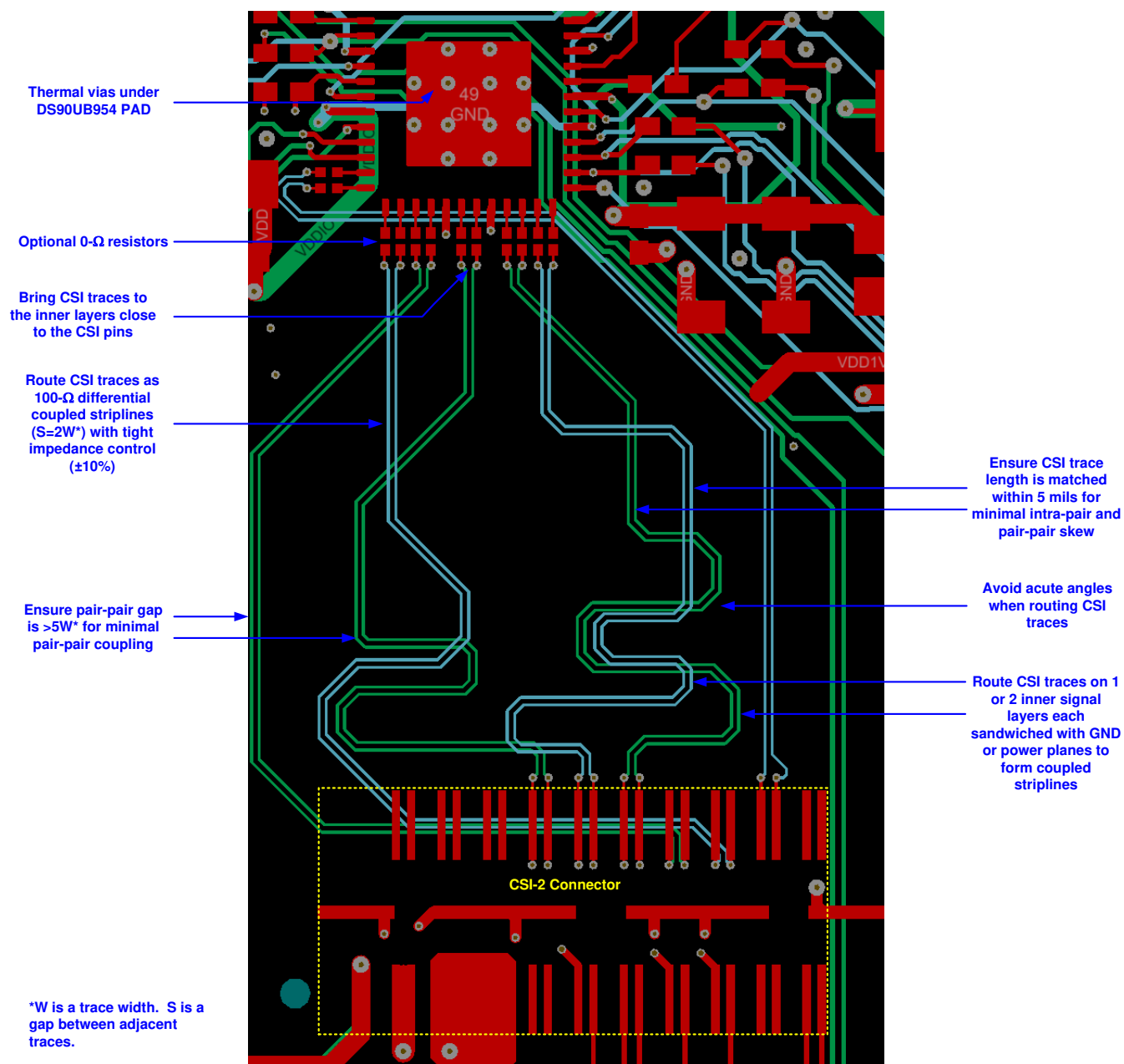
FIG 10-3. DS90UB954-Q1 PCB Layout Example: CSI-2 Traces
