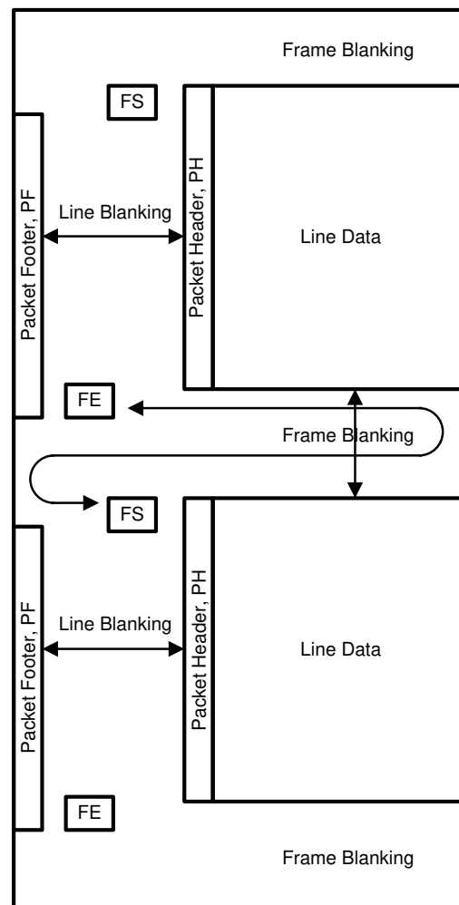
FIG 6-9. CSI-2 General Frame Format
