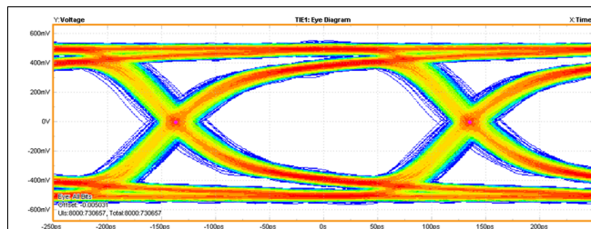
図 8. DOUT0 Eye at 3.675 Gbps
