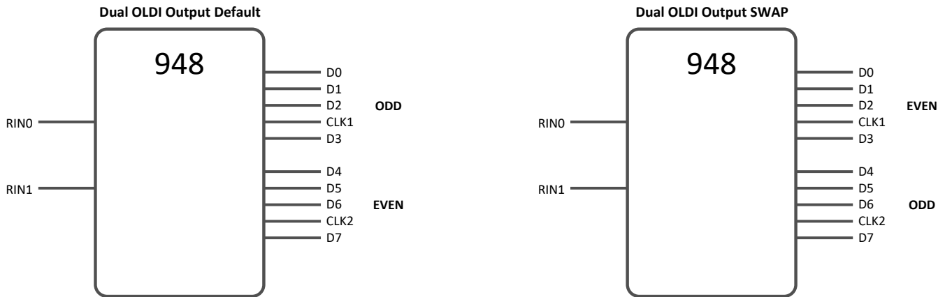
図 7-17. Dual oLDI Output SWAP
