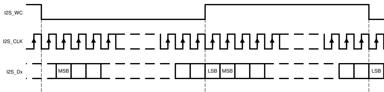
図 8-8. I2S フレームのタイミング図
