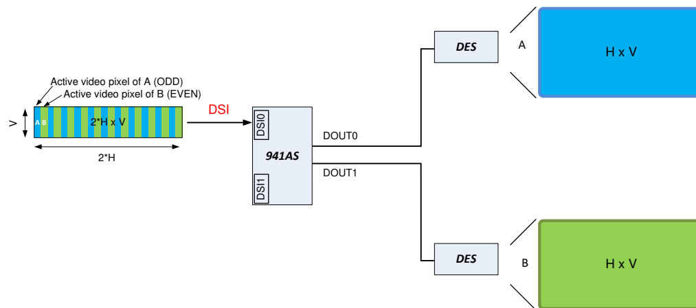
図 8-24. 交互ピクセル分割
