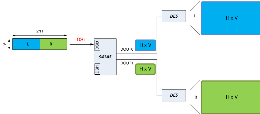
図 8-15. シリアルライザで分割する方法
