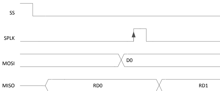
図 8-6. リバース・チャネル SPI 読み出し
