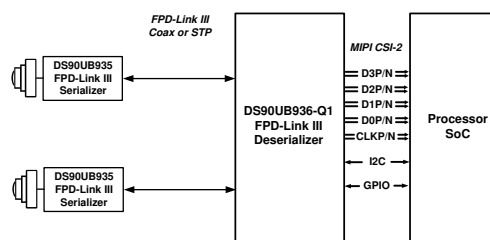
代表的なアプリケーション回路図
