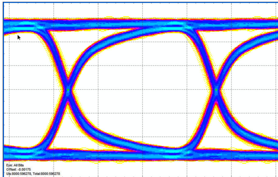
図 5-3. FPD-Link III フォワード チャネル (シリアル出力) のアイ ダイアグラム垂直スケール: 100mV/DIV、 水平スケール: 100ps/DIV
