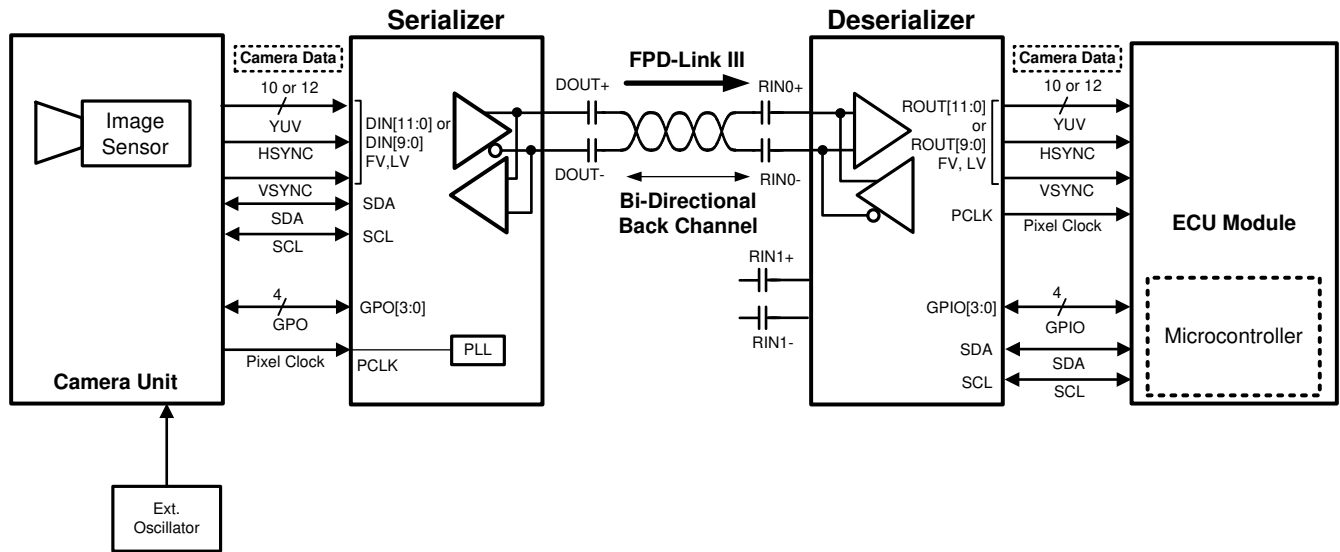
図 7-5. DS90UB933-Q1/934-Q1 Operation in PCLK mode
