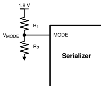
図 7-6. MODE Pin Configuration on DS90UB933-Q1
