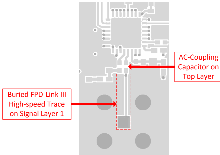
図 10-2. DS90UB933-Q1 Serializer DOUT+ Trace Layout
