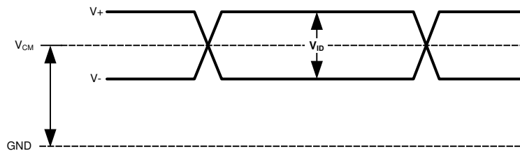
FIG 6-2. FPD-Link Receiver VID
