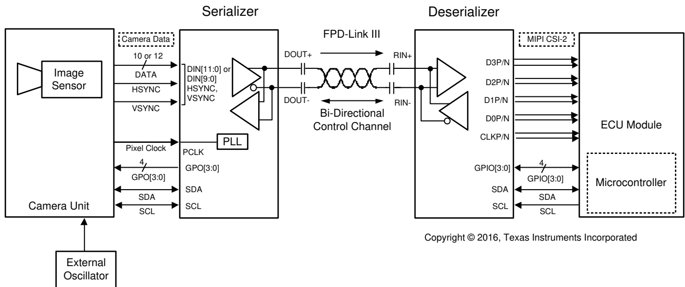
7-5. DS90UB633A-Q1/662-Q1 Operation in PCLK mode
