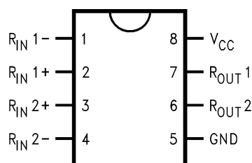
接続図
