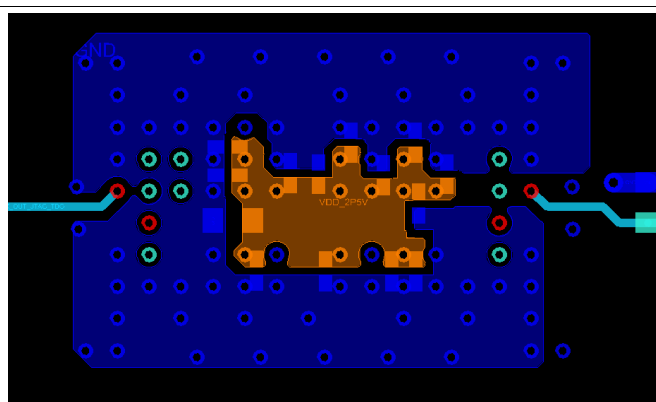
图 38. Microstrip Example, Bottom Layer
