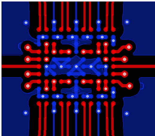
図 25. Top Layer
