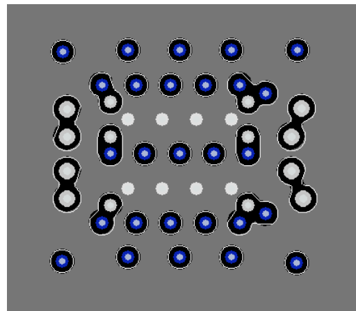
図 28. VDD Layer
