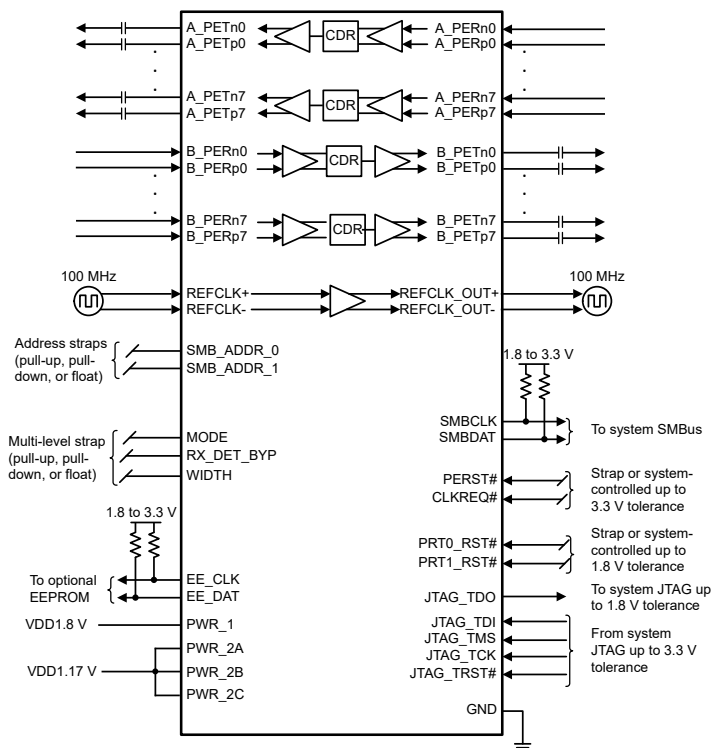
概略回路図
