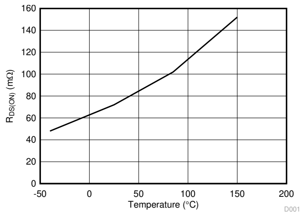
图 6-2. R_{DS(on)} vs Temperature
