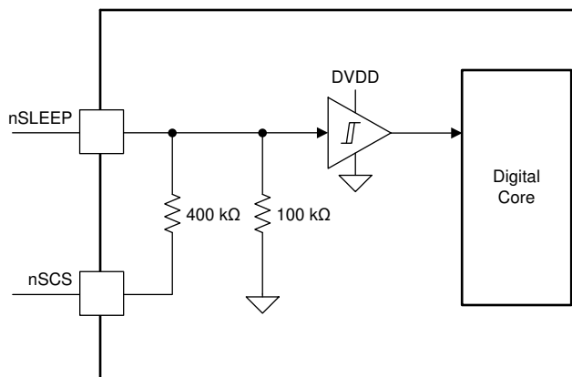
图 7-11. nSCS and nSLEEP Circuit
