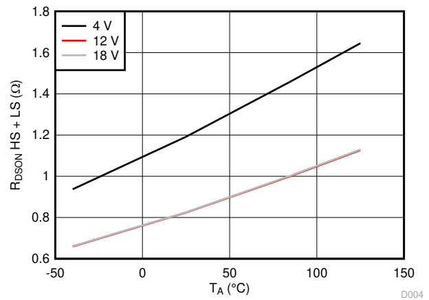
図 5-4. R_{DS(on)} vs Temperature
