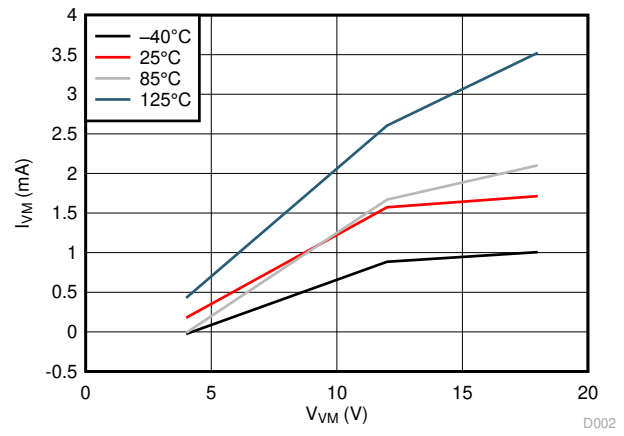
図 5-2. I_{VMQ} vs V_{VM}
