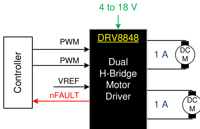
概略回路図
