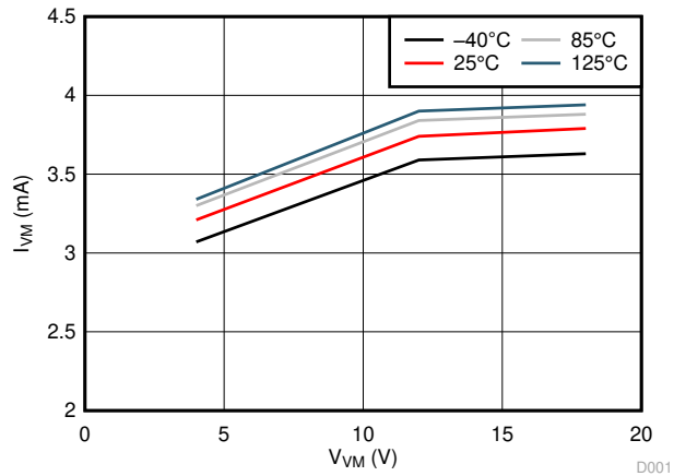
図 5-1. I_{VM} vs V_{VM}
