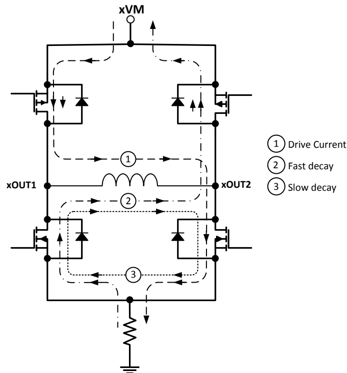
图 6-3. Decay Modes
