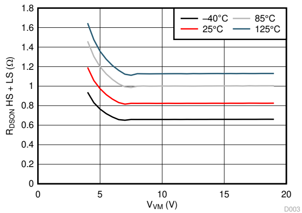
図 5-3. R_{DS(on)} vs V_{VM}
