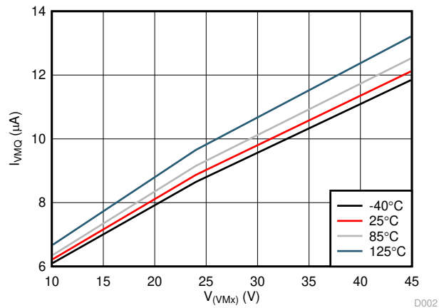
6-2. I_{VMxQ} vs V_{VMx}
