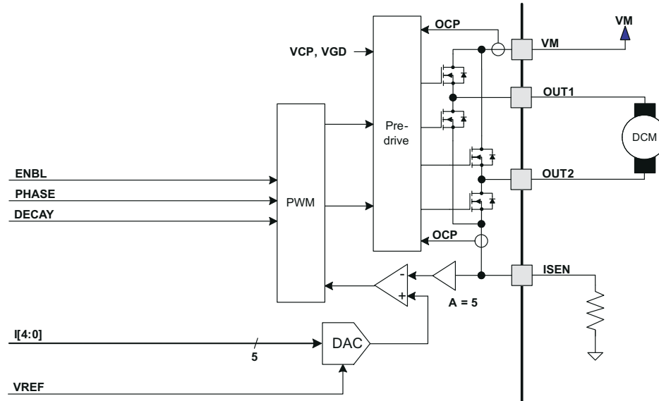
図 7-1. Motor Control Circuitry
