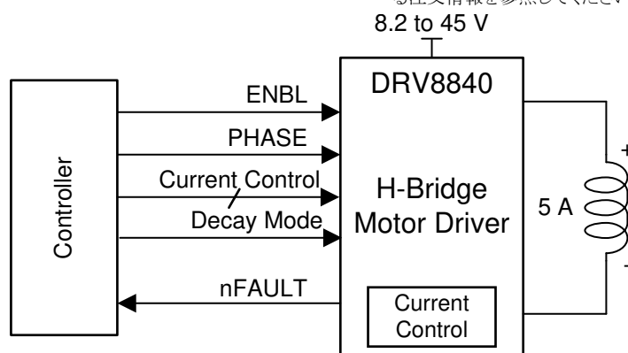
簡略回路図
