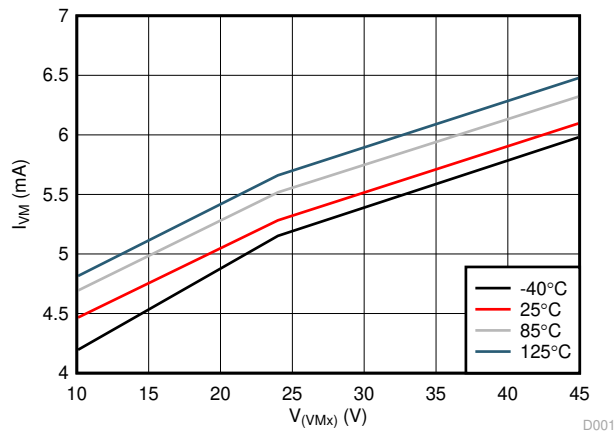
6-1. I_{VMx} vs V_{VMx}
