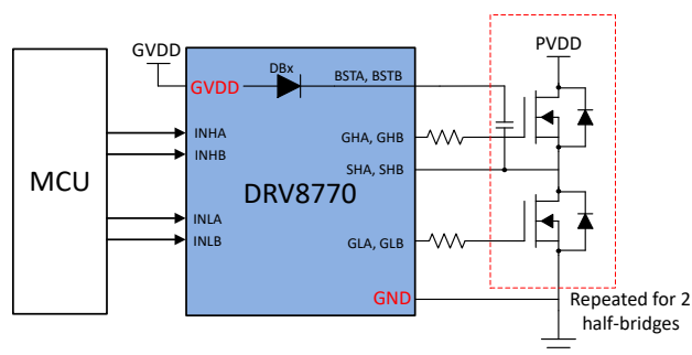
概略回路図 (DRV8770)
