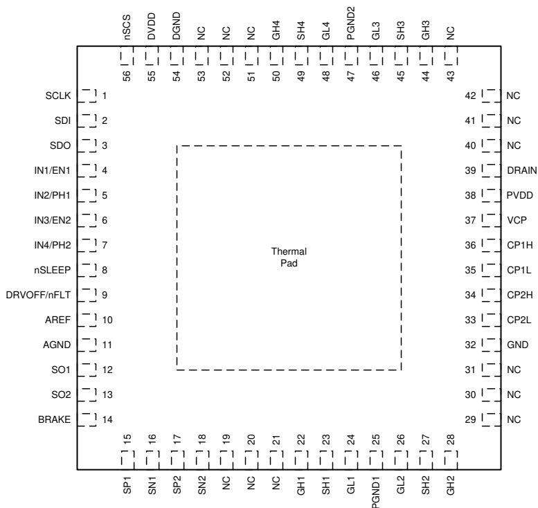
図 5-2. DRV8714S-Q1 VQFN (RVJ) 56-Pin Package Top View
