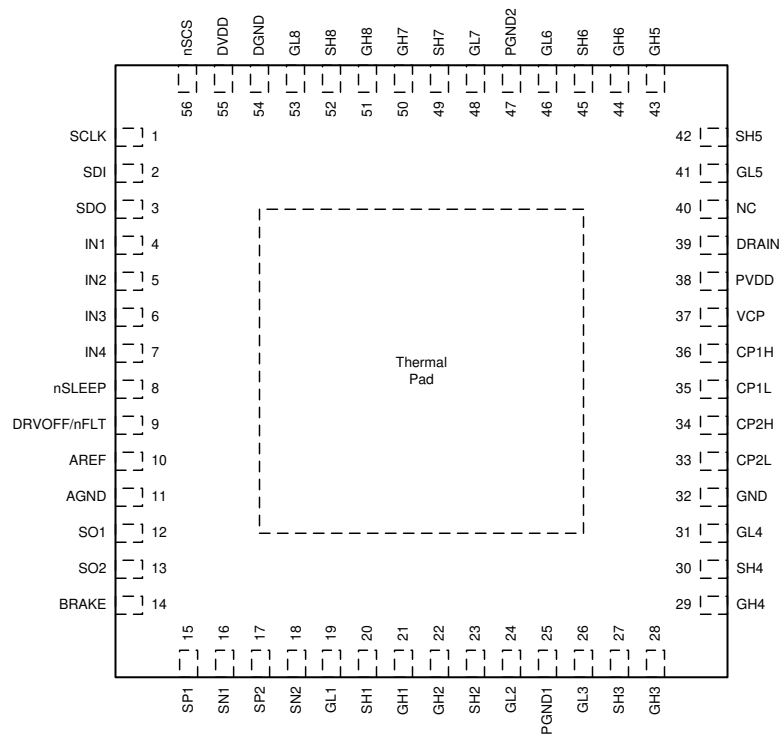
図 5-1. DRV8718S-Q1 VQFN (RVJ) 56-Pin Package Top View
