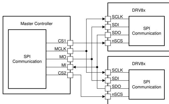
図 6-21. デジタイズ・チェーンを使わない SPI 動作
