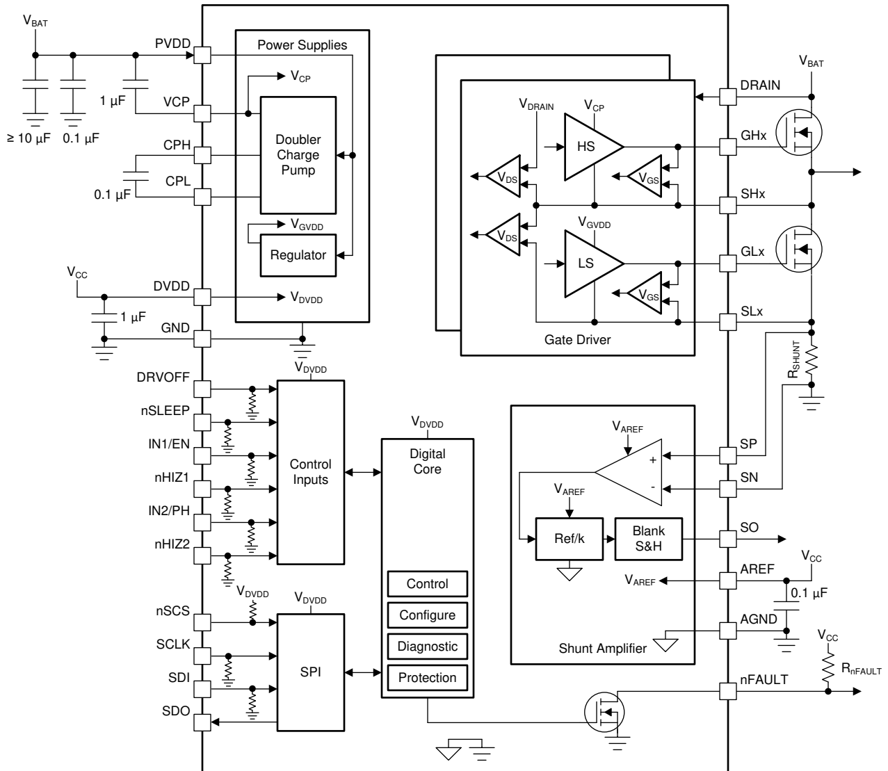
図 6-1. DRV8705S-Q1 の機能ブロック図
