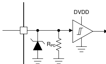
図 6-13. 入力ピンの構造
