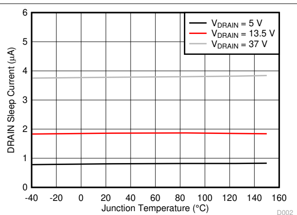
図 5-3. DRAIN スリープ電流
