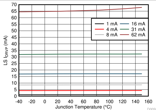
図 5-10. ローサイド・ゲート・ドライバ・ソース電流
