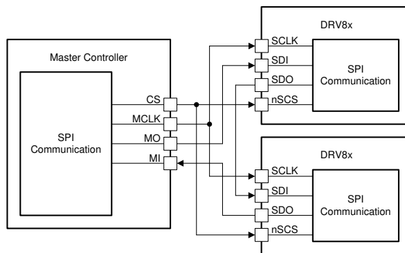
図 6-22. デジタイズ・チェーンを使った SPI 動作
