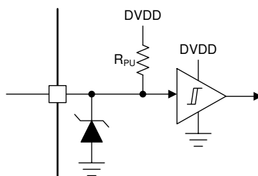
図 6-14. 入力ピンの構造 (nSCS)
