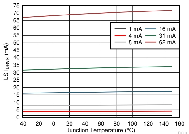
図 5-11. ローサイド・ゲート・ドライバ・シンク電流
