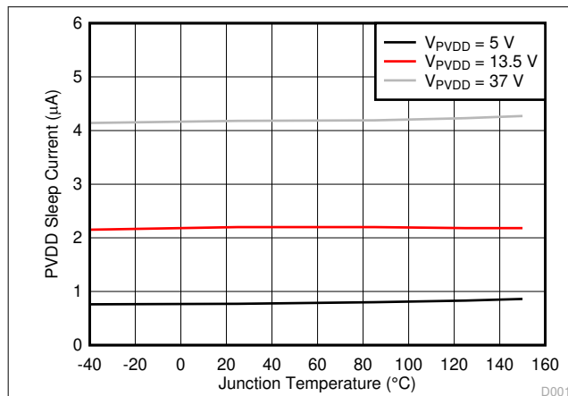
図 5-2. PVDD スリープ電流
