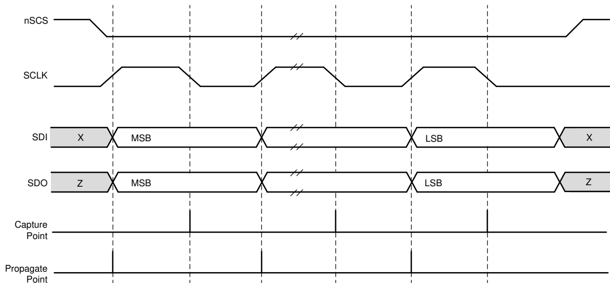
图 7-18. SPI Transaction
