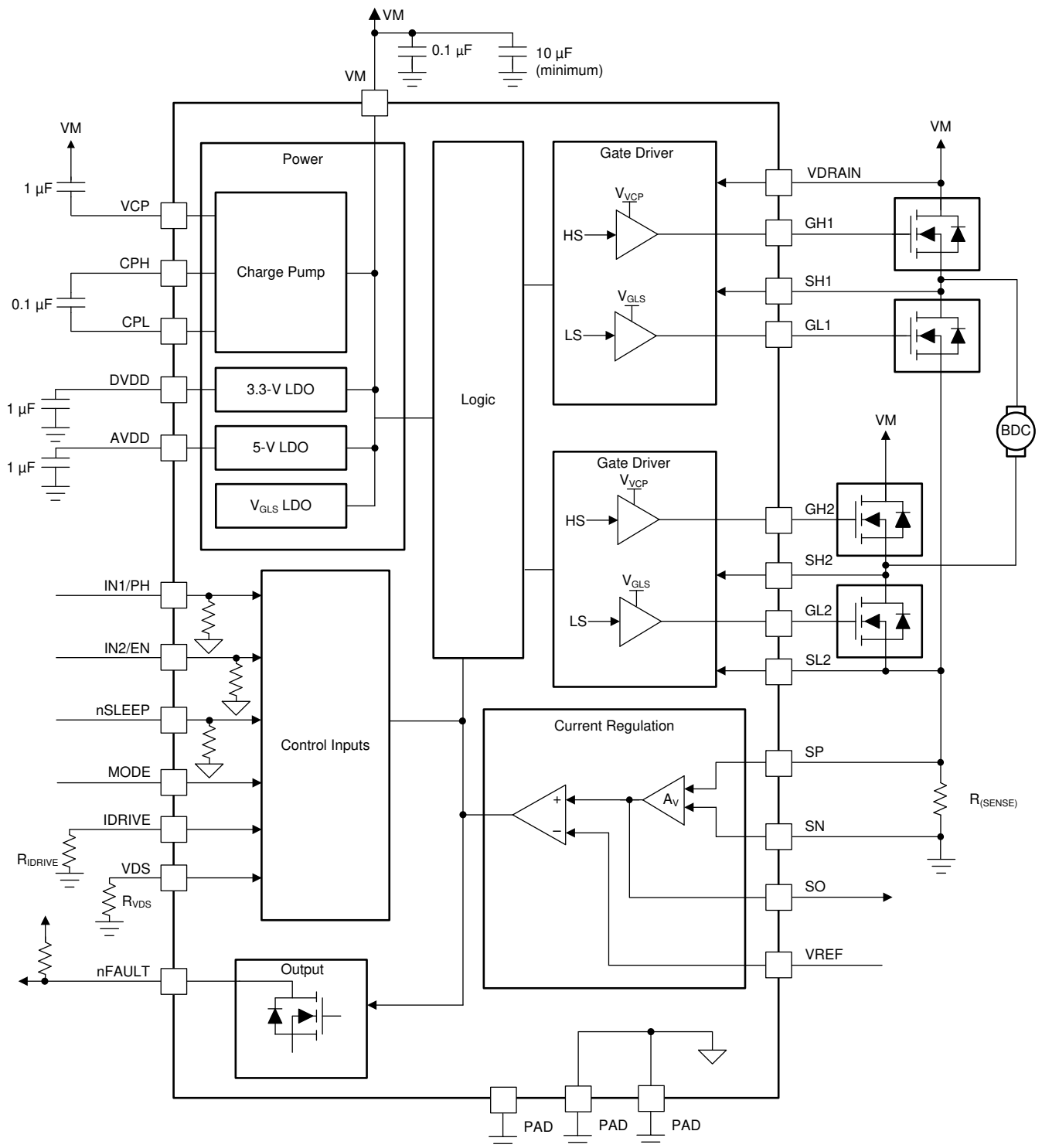
図 7-1. DRV8702-Q1 Functional Block Diagram
